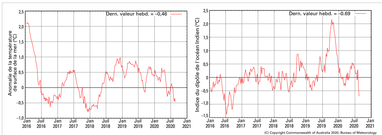
Figure 5. Valeurs de l'indice Niño 3.4 de la température de surface de la mer (à gauche) et de l'indice du dipôle de l'océan Indien (à droite) de 2016 au début de 2020 Source: Service météorologique australien (BoM)
