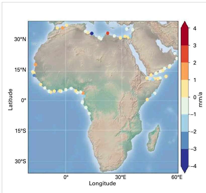
Figure 10. Écart dans les variations du niveau de la mer entre la zone côtière (0 – 4 km) et le large (15 km). Les points rouges/bleus signalent les tendances côtières supérieures/inférieures à celles du large. À noter l'absence d'écart notable dans de nombreux cas. Source: LEGOS, France
