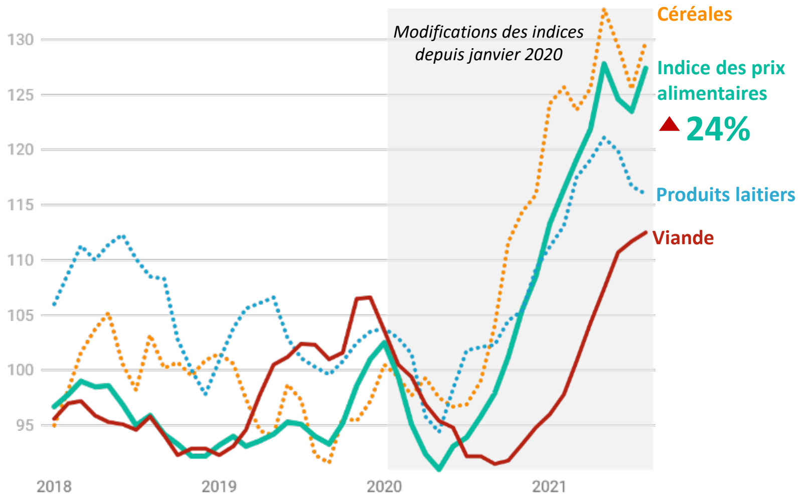
Indices mondiaux des prix alimentaires, 2018-août 2021
